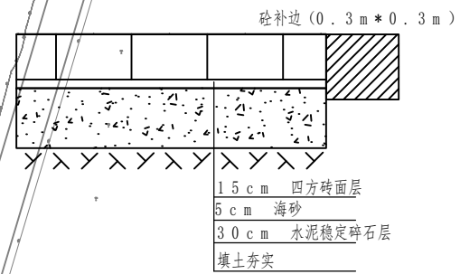
四方砖面层断面图
