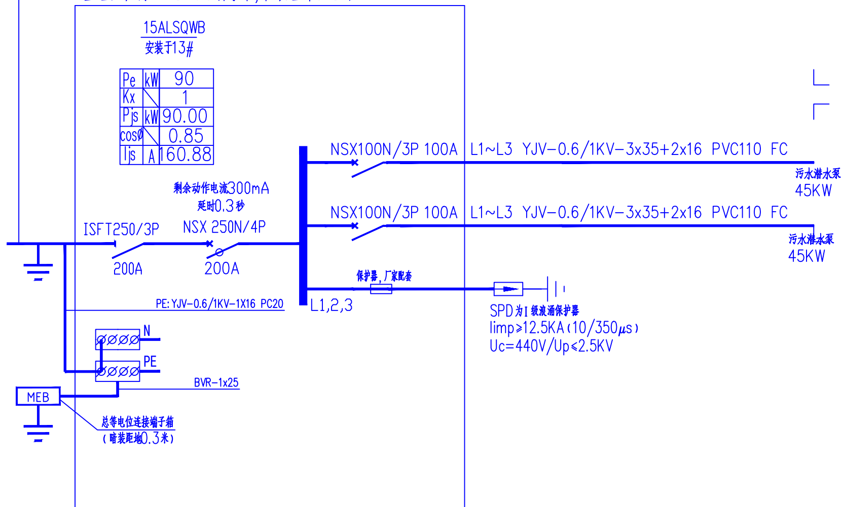
15ALSQWB 配电箱系统图
