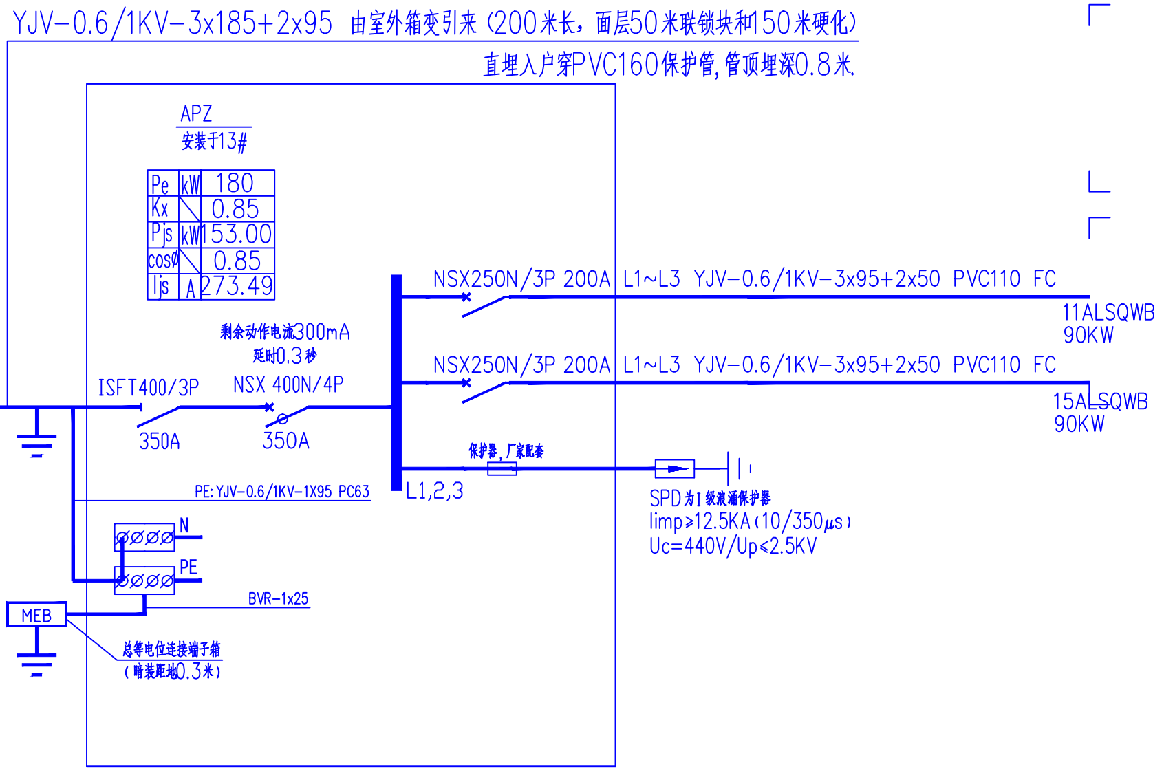
APZ 总配电箱系统图
