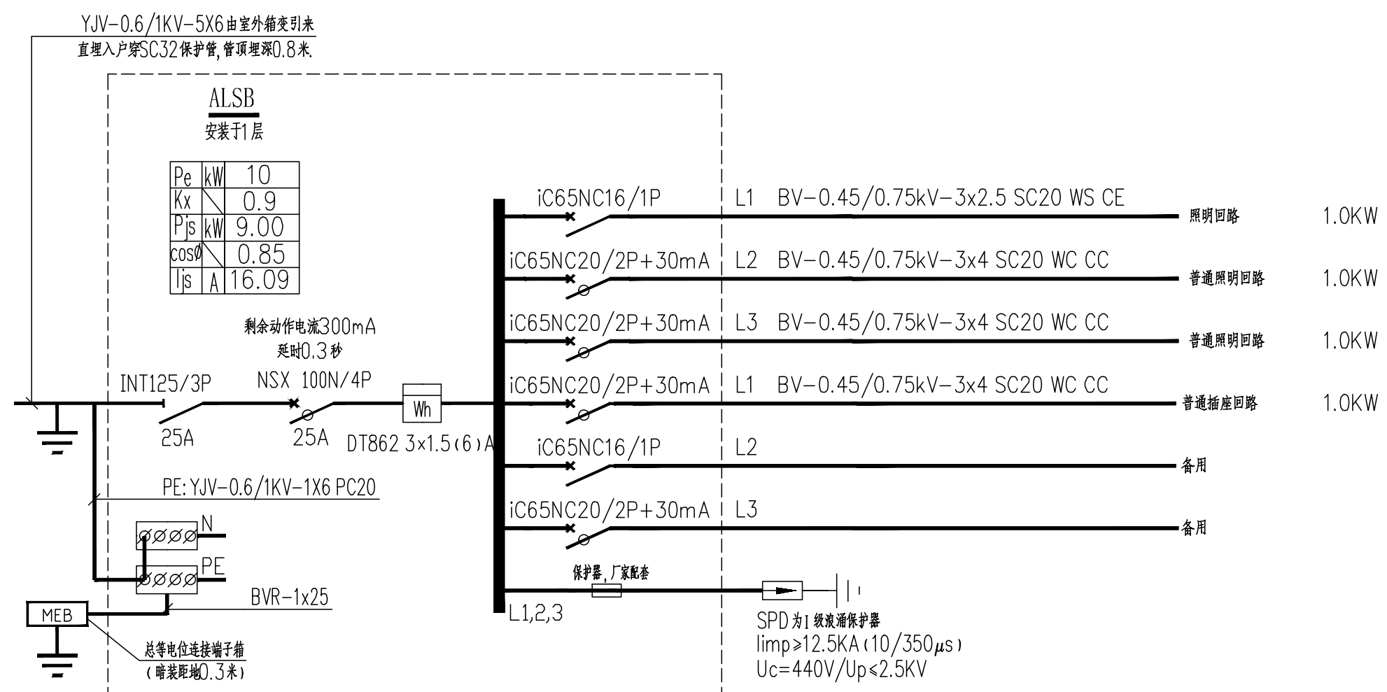
ALSBS总配电箱系统图
