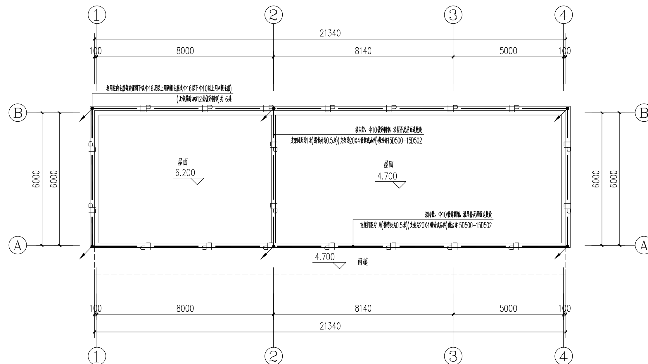
屋顶层防雷平面图 1:100
